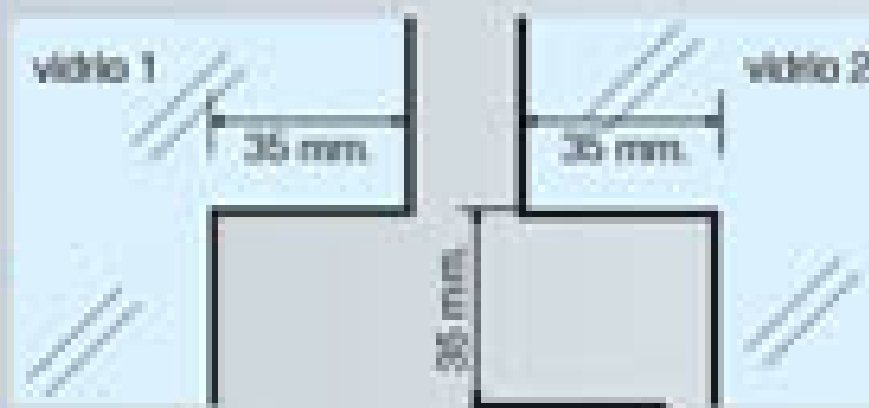
medidas de corte en vidrios
