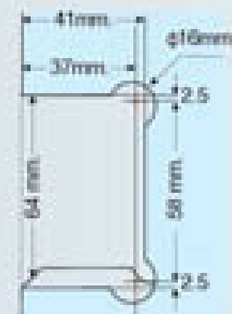
Saque o corte en vidrio
