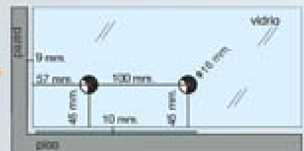
medidas de perforado en vidrios para TMZ-TI26
