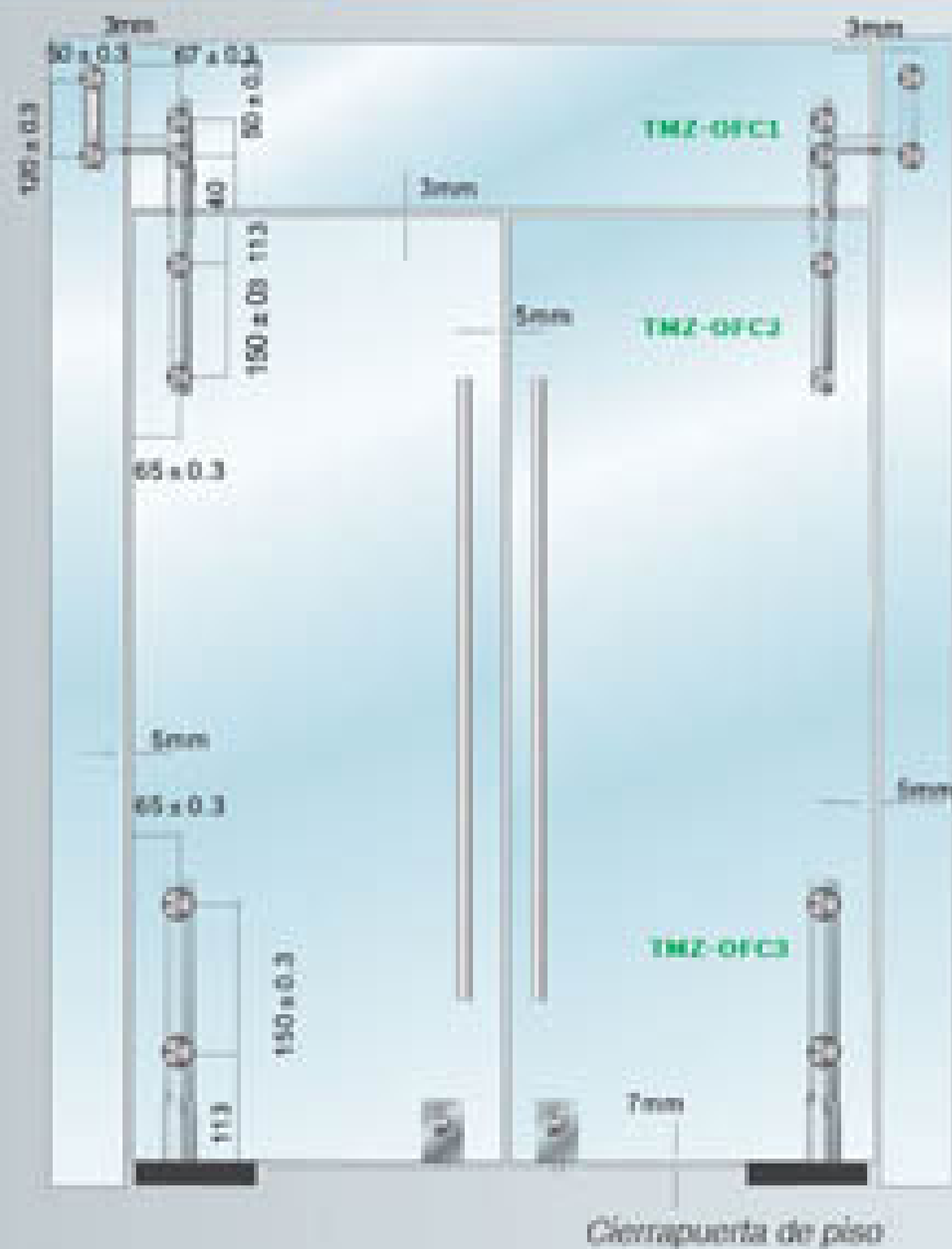
Ejemplo de mampara [E]
