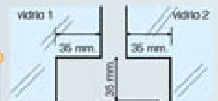
medidas de corte en vidrios
