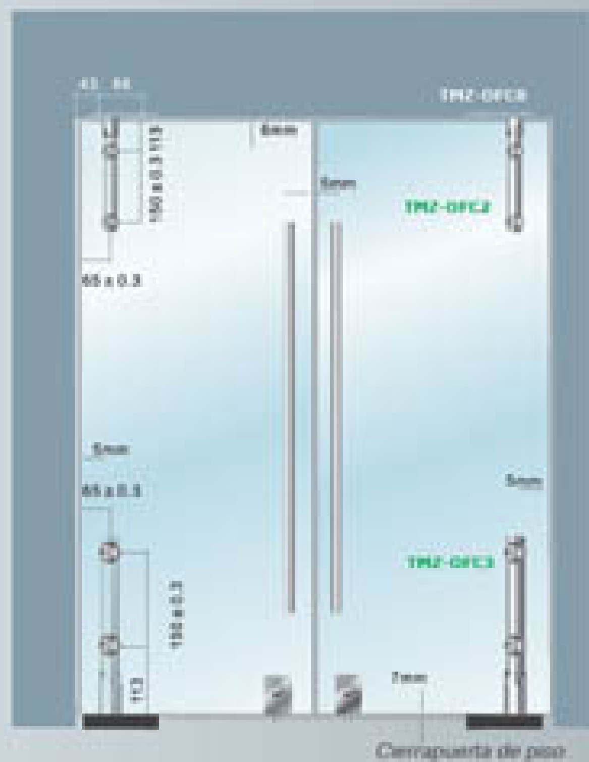
Ejemplo de mampara [D]
