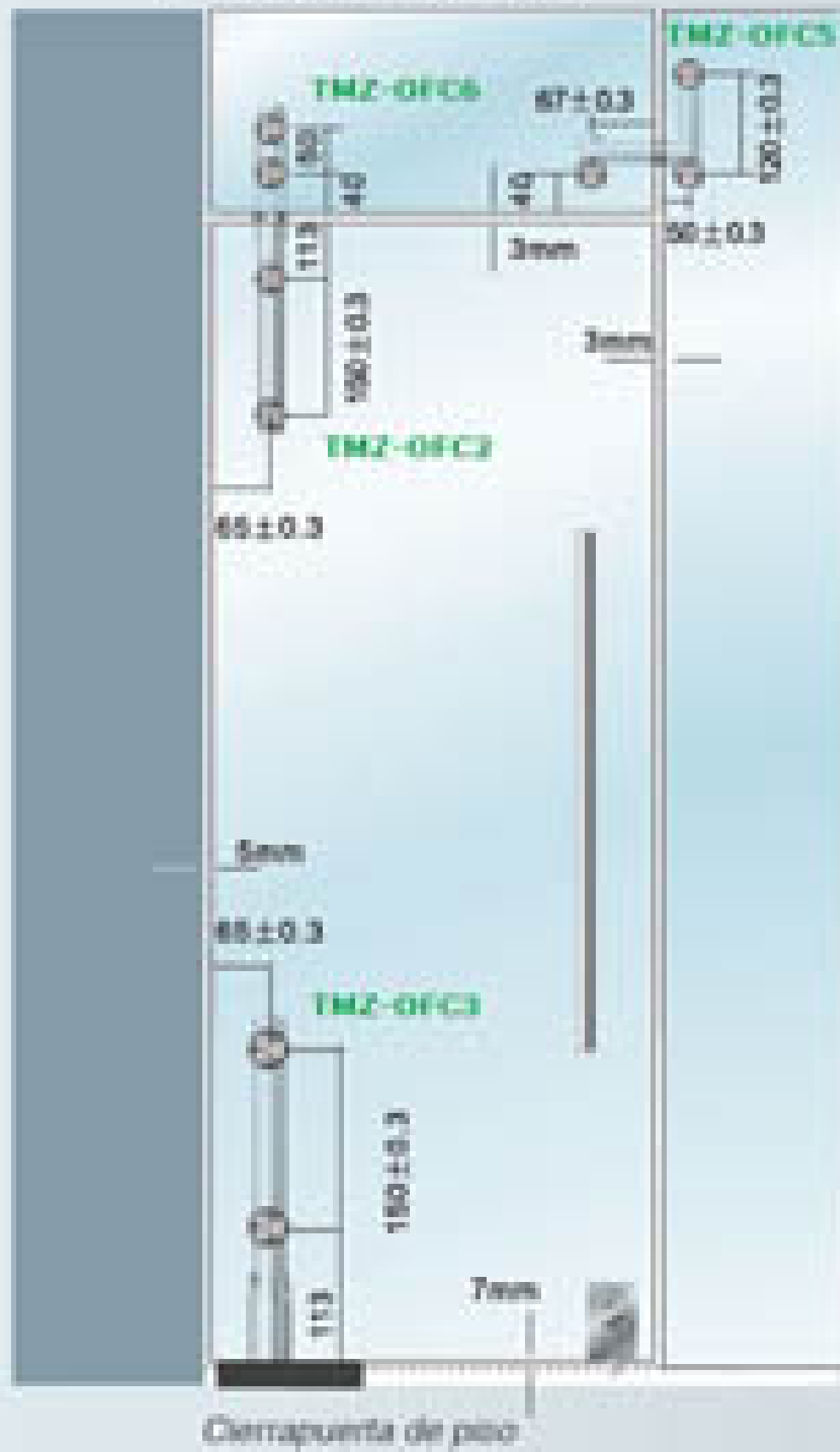
Ejemplo de mampara [A]
