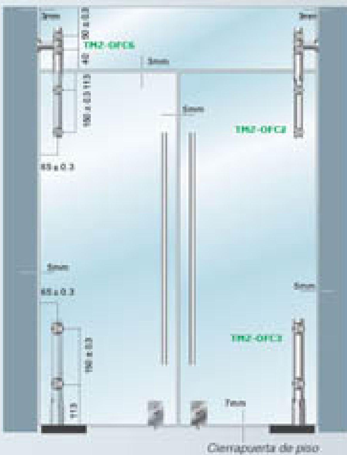
Ejemplo de mampara [C]
