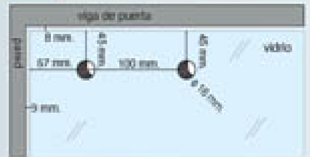
medidas de perforado en vidrios para TMZ-TP28
