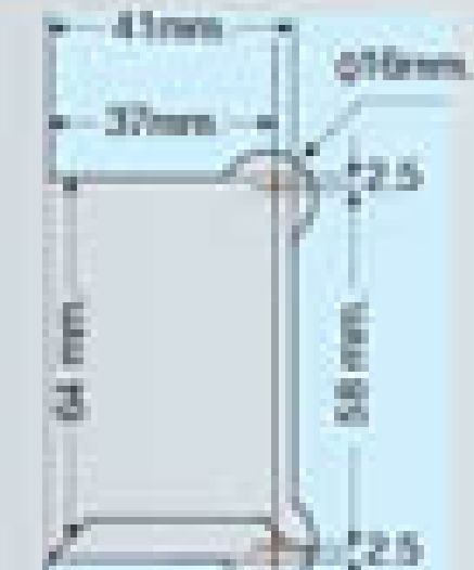
Saque o corte en vidrio
