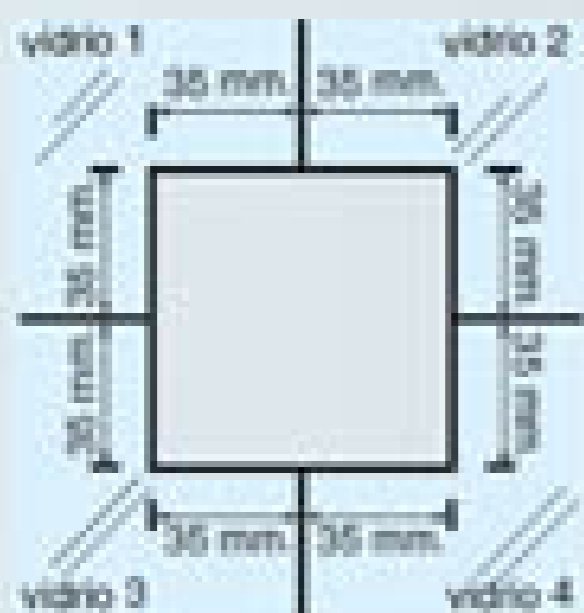
medidas de corte en vidrio
